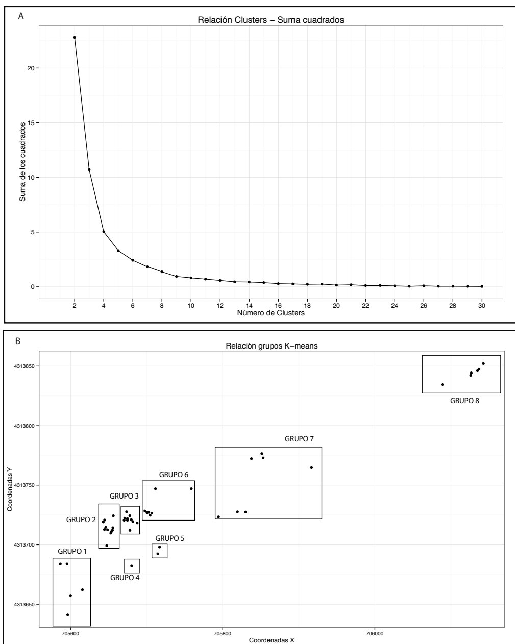
Fig. 23. Resultados del test K-means.
