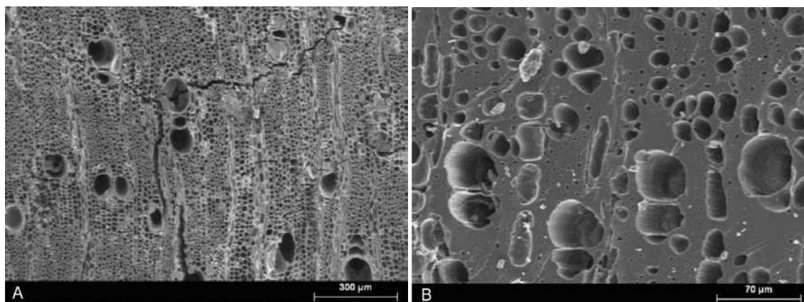
Fig. 8. A, plano transversal de Ficus carica procedente de Q057 (x80); B, plano transversal de Olea europaea vitrificado recogido en Q077 (x350).
