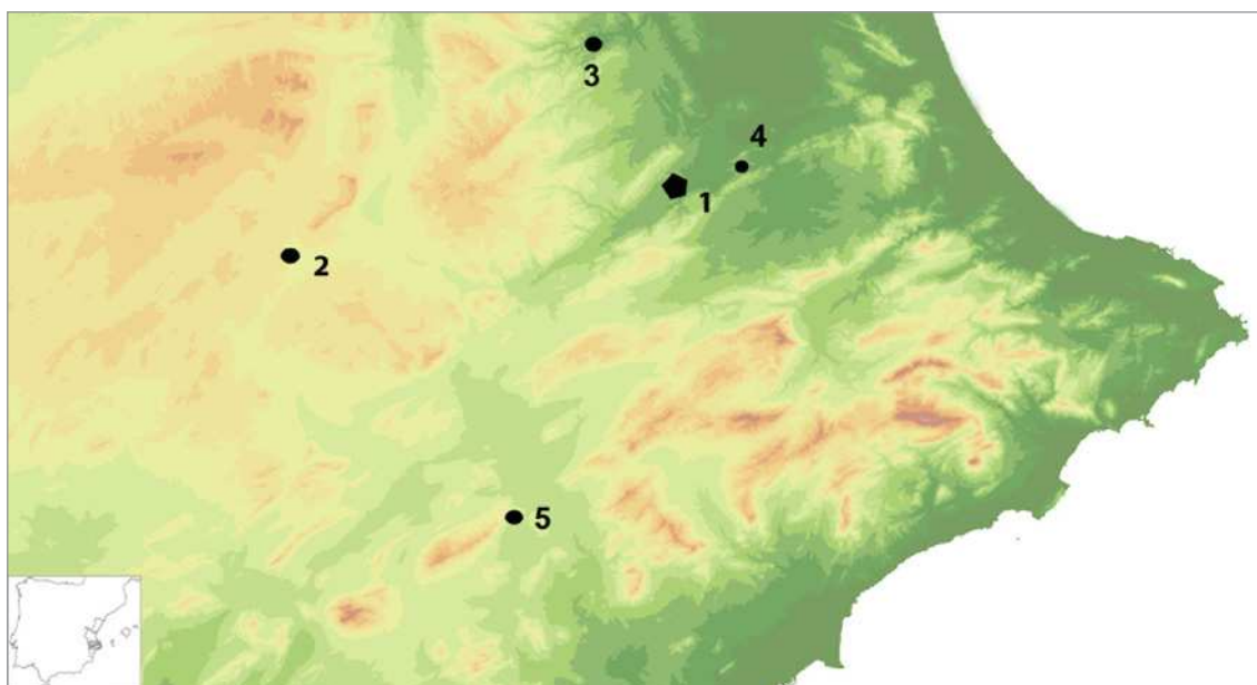
Fig. 19. Mapa de localización de emplazamientos de diabasas. 1, situación de Quintaret; 2, Cerro del cuchillo (Almansa); 3, Quesa; 4, Lloc Nou de Fenollet; 5, depresión del Vinalopó.
