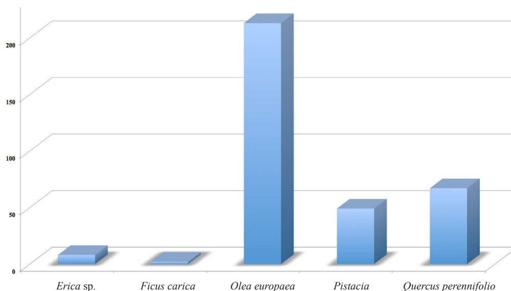
Fig. 7. Representación de los diferentes taxones dentro de la muestra antracológica recuperada en las estructuras calcolíticas de Quintaret.
