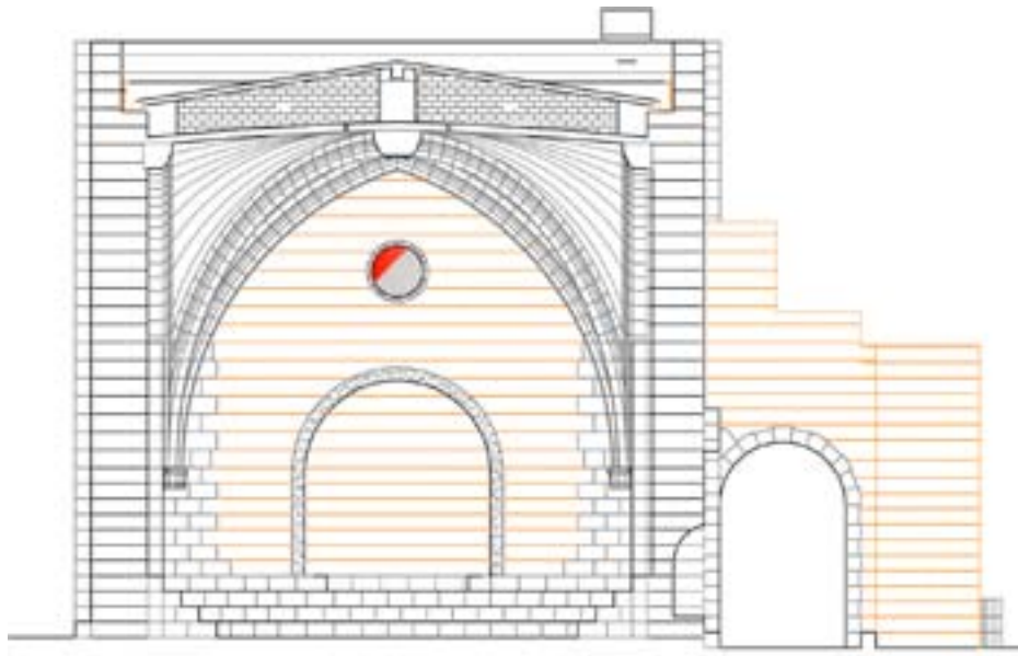
Secció est
